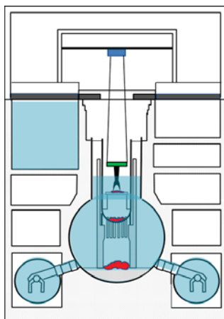
a. 冠水-上アクセス工法
