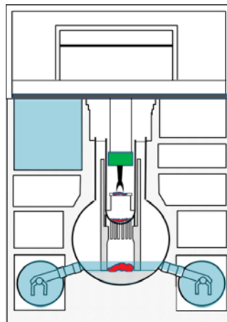
b. 気中-上アクセス工法
