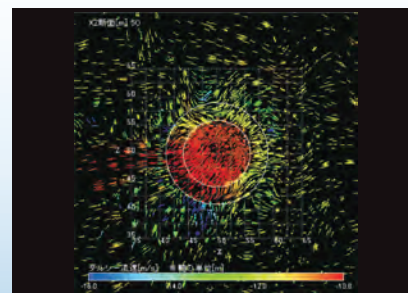
地中に埋設した際の地下水との関係のシミュレーション結果 Simulation results of the relationship between groundwater and high-level waste
