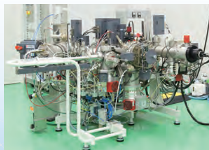
二重収束型二次イオン質量分析装置(CAMECA IMS 7f-Auto) Dynamic Secondary Ion Mass Spectrometer
