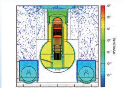
原子炉建屋内部の放射線量率シミュレーション Simulation result of dose rate distribution inside the reactor building
